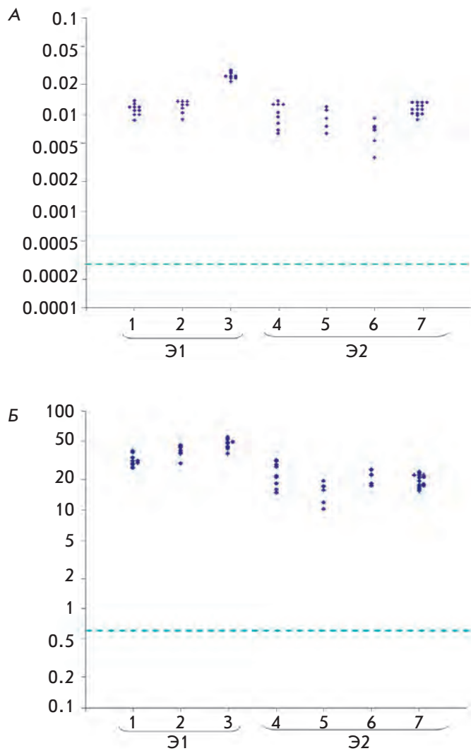
Рис. 2. Содержание (А) и концентрация (Б) ^{110m}\text{Ag} -НЧ серебра в плодах крыс. Ось абсцисс – № беременной самки, № эксперимента; ось ординат – содержание НЧ, % от введенной дозы (А), концентрация НЧ (нг/г образца) (Б). Здесь и на рис. 3 пунктиром показан предел количественного определения ^{110m}\text{Ag} -НЧ в образцах
