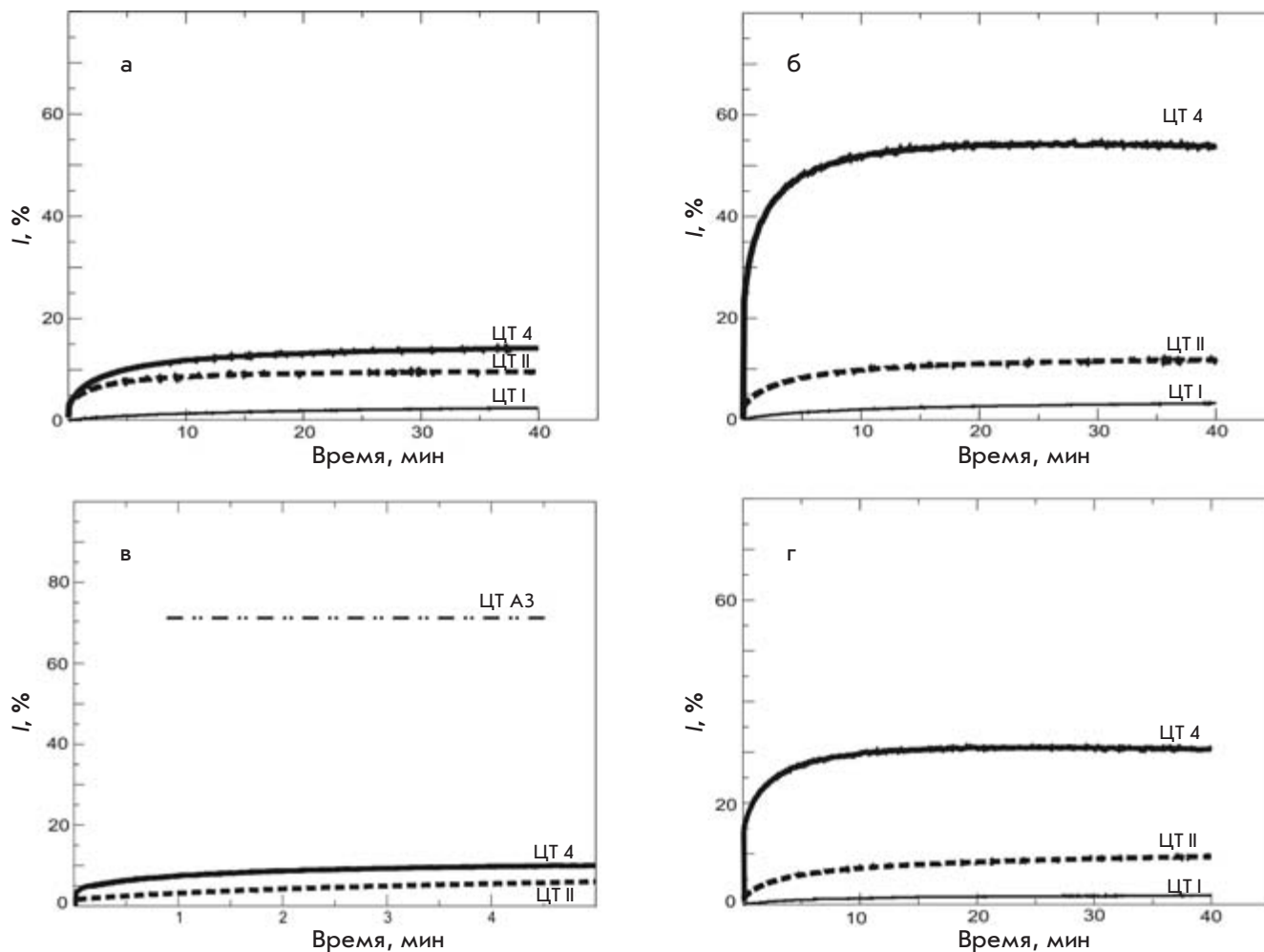
Рис. 2. Интенсивность вытекания флуорофора (кальцеин) из липосом состава ПОФХ (а), ПОФХ/ФС5% (б) и ПОФХ/Сф5% (г) в присутствии ЦТ I, ЦТ II ( N. oxiana ) и ЦТ 4 ( N. kaouthia ). в – Кинетика флуоресценции карбоксифлуоресцеина (6-CF) в первые минуты после добавления ЦТ 4 и ЦТ II. В данном эксперименте (в) состав буфера, флуоресцентный краситель, соотношение L/P = 62.5 и концентрация липид/токсин (10/0.16 мкМ) в измеряемом объеме повторяют условия работы [6]. Интенсивность флуоресценции 6-CF при действии ЦТ АЗ ( N. atra ), зарегистрированная в работе [6], отмечена ( _ _ _ ).
